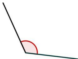
stumpfer Winkel
