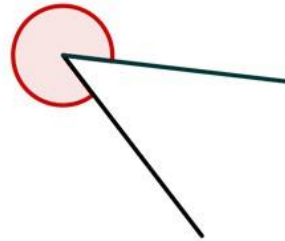
erhabener Winkel
